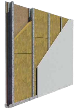
Muros de paneles de yeso de capa sencilla o multicapa con clasificación UL.
